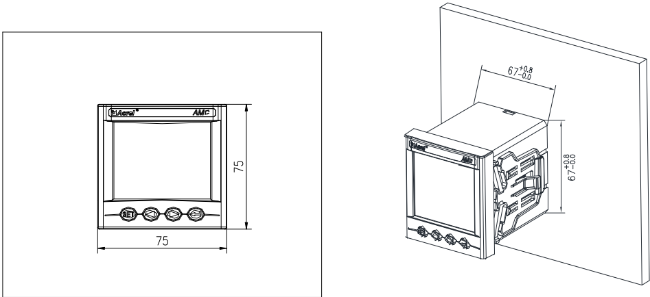
图 3 AMC72 安装尺寸
